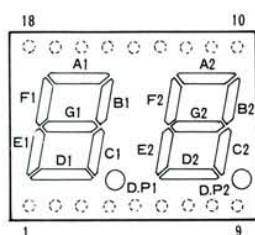
GL7S201J(DS101)
