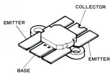
2SC2630(Q902)
