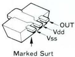
RH5VA32AA (D5) (Q2021)
