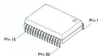
TD62C850N(Q101)
