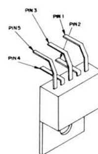
TDA2003H(Q1023)
