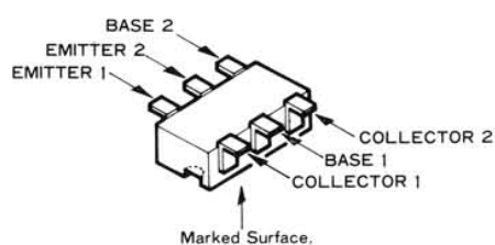
IMH5(H5)(Q2003)
