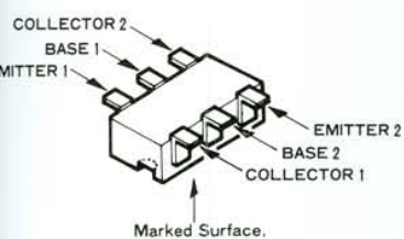
IMD2(D2)(Q2010)
