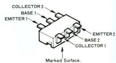
IMD2(D2)(Q2010)
