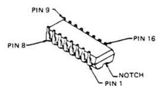
MC3361P(Q1008)
